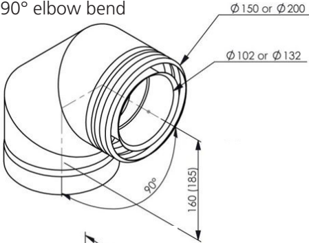
11 USB 90 100 (Ø100) USB 90 130 (Ø130) 90° elbow bend
