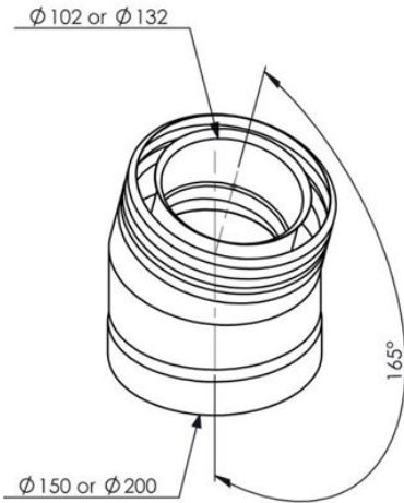
13 USB 15 100 (Ø100) USB 15 130 (Ø130) 15° elbow bend
